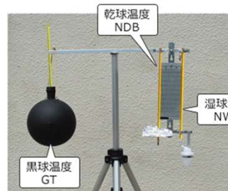
暑さ指数(WBGT)測定装置
